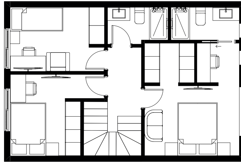
PLANTA ALTA
